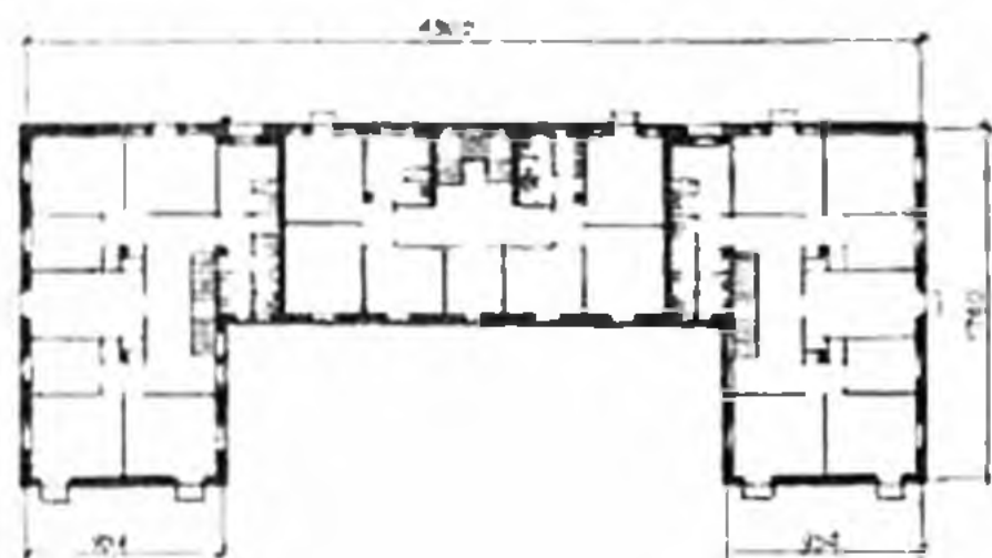
Общезитие на 130 человек. Авторы — член-корреспондент Академии архитектуры СССР Е. А. Левинсон и арх. Л. Е. Асс. План 2-го этажа.
