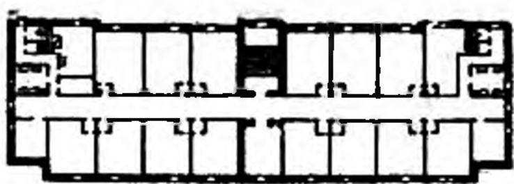
Общежитие на 150 человек. Автор арх. А. Е. Катонин. План 2-го этажа
