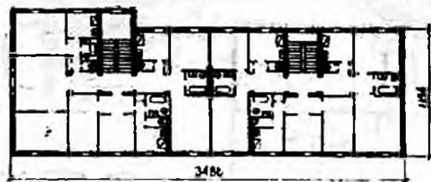
Жилой дом. Автор арх. Б. С. Эбарж. План 2-го этажа.
