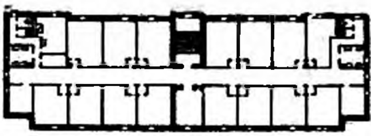
Общежитие на 150 человек. Автор арх. Л. Е. Катонина. План 2-го этажа
