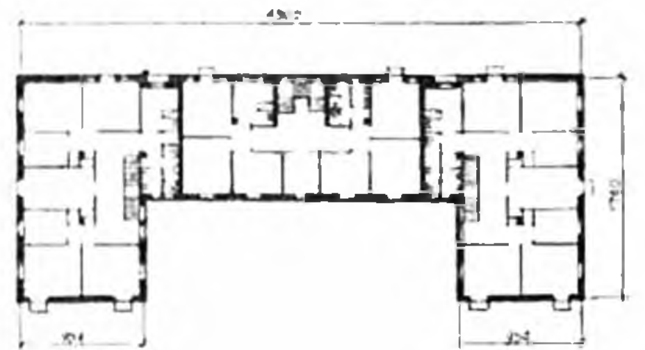
Общедомовое на 130 человек. Авторы — член-корреспондент Академии архитектуры СССР Е. А. Левинсон и арх. Л. Е. Асс. План 2-го этажа.
