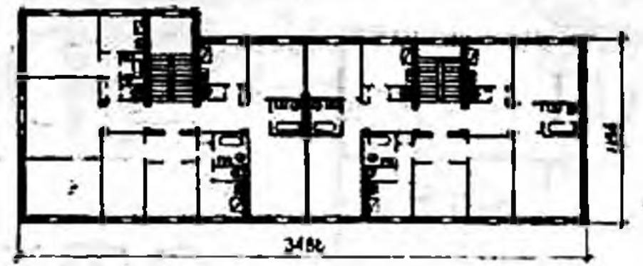
Жилой дом. Автор арх. Б. С. Эбарж. План 2-го этажа.
