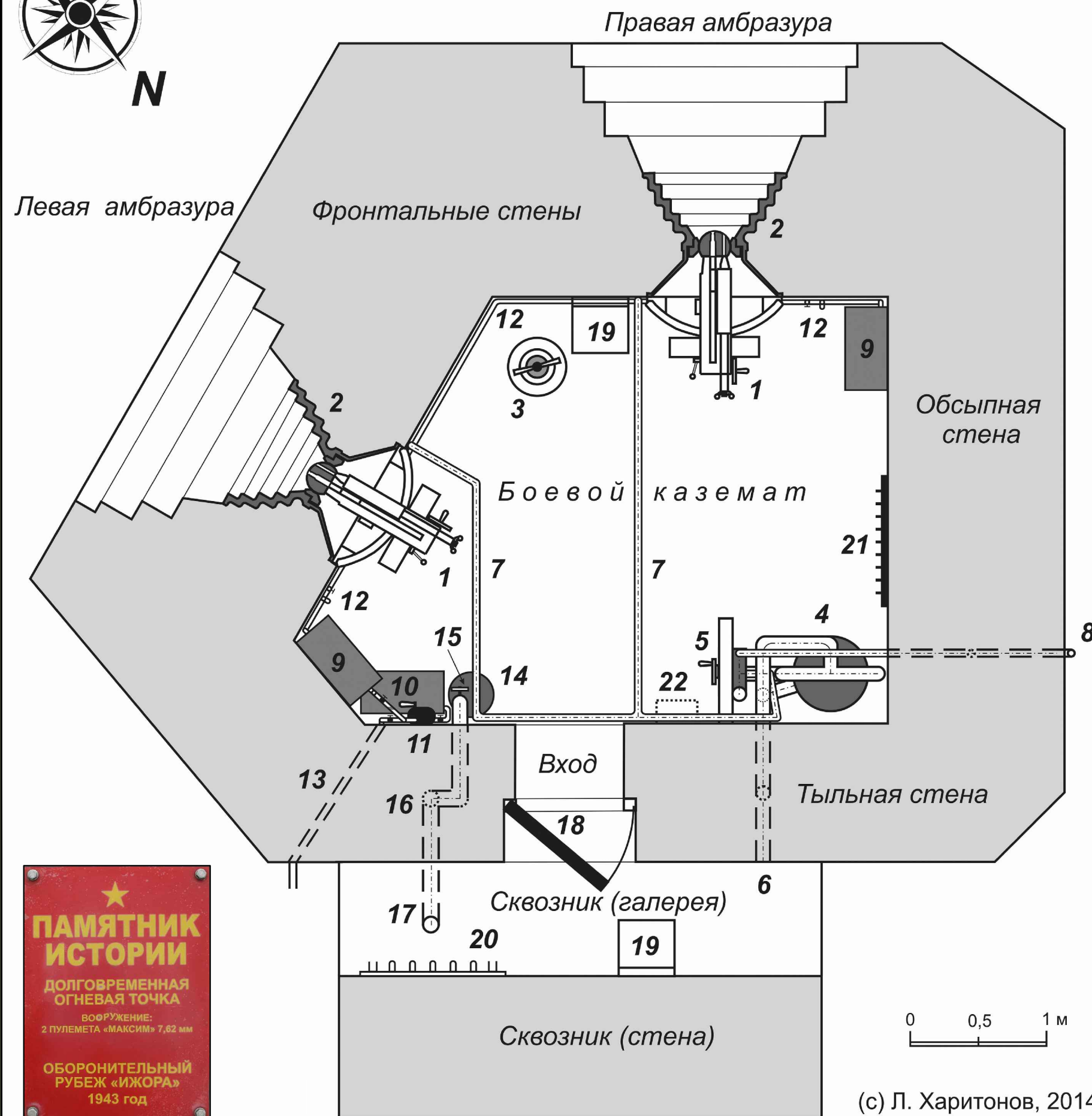
Схема сооружения.
